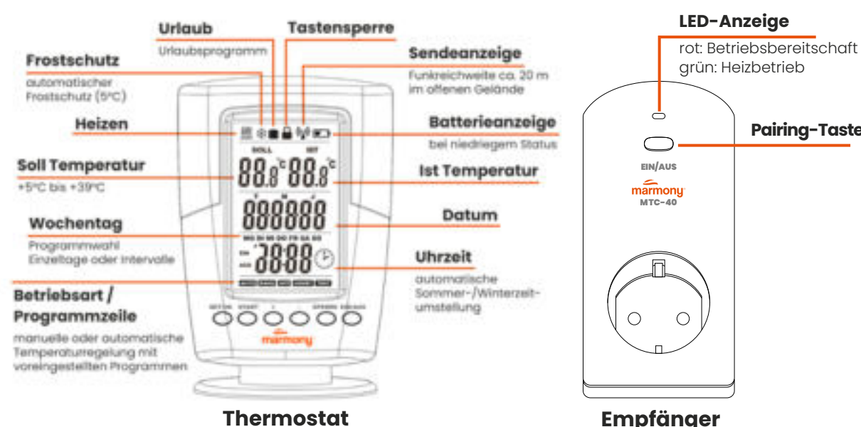
Abb. 08: Thermostat und Empfänger
