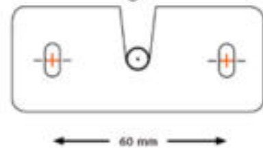
Abb. 03: Bohrlöcher
